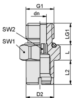
Конструктивные данные SC-A 045 M16-AG L
