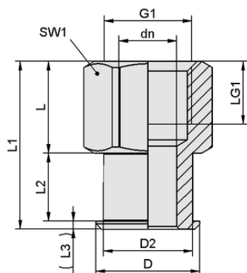
Конструктивные данные SC 090 G3/8-IG
