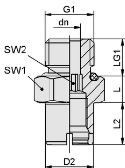
Données de construction SC-A 045 M12-AG L
