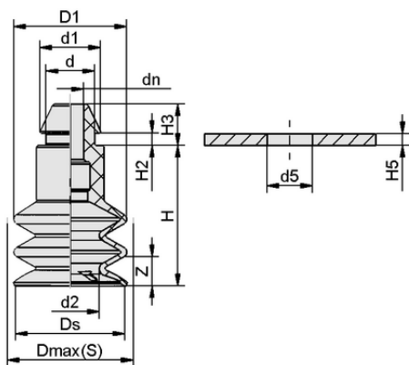
Конструктивные данные SAB2 20 HT1-60 P
