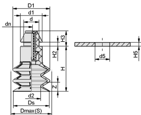
Dati di costruzione SPB2 20 SI-40 SW100 P
