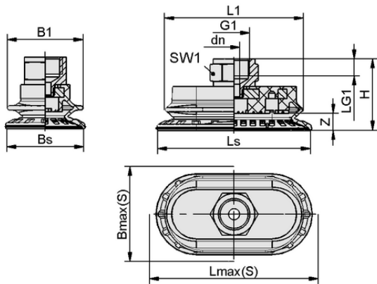
Datos de diseño SAOB 140x70 HT1-60 G3/8-IG
