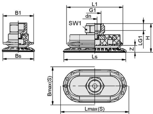
Datos de diseño SAOB 80x40 HT1-60 G3/8-IG
