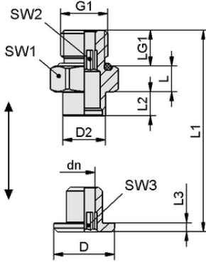
Tasarım verileri SC 065 G1/4-AG L MOD
