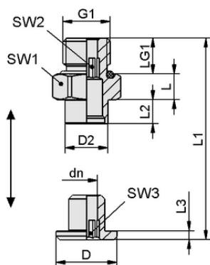
Конструктивные данные SC 065 G1/4-AG L MOD
