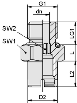
Tasarım verileri SC-A 045 M12x1.5-AG L
