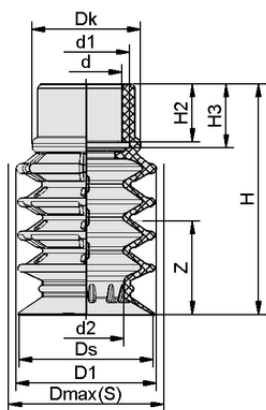
Конструктивные данные SPB4 30 SI-HD-65 SC080
