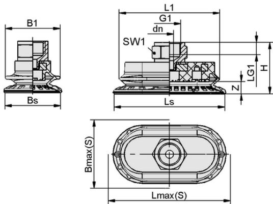
Données de construction SAOB 80x40 HT1-60 G1/4-IG
