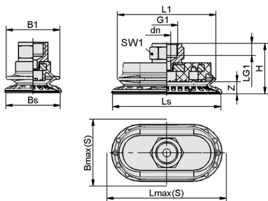
Datos de diseño SAOB 80x40 HT1-60 G1/4-IG
