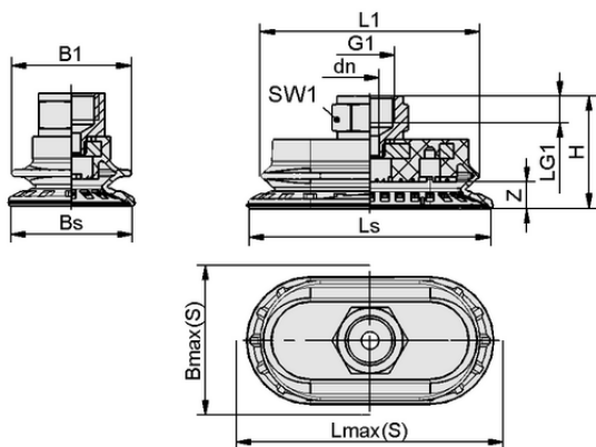
Design data SAOB 60x30 HT1-60 G1/4-IG
