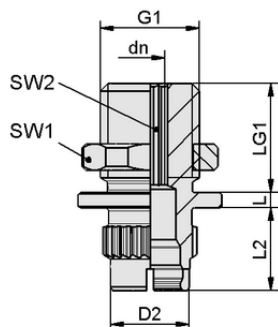
Конструктивные данные SC-A 055-AR M14x1.5-AG L
