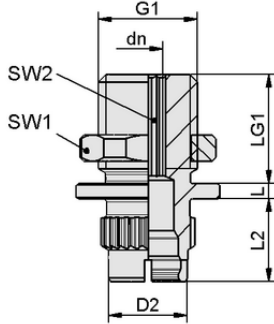
Tasarım verileri SC-A 055-AR M10-AG L
