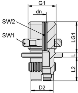
Tasarım verileri SC-A 055-AR G3/8-AG L
