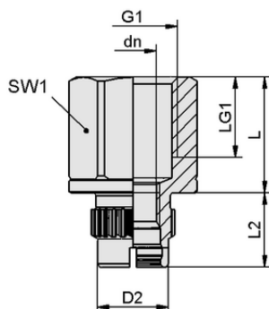
Dati di costruzione SC-A 055-AR G3/8-IG L
