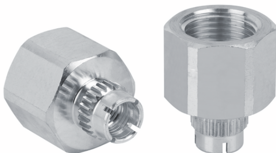
SC-A 055-AR G3/8-IG L
