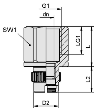
Design data SC-A 055-AR G3/8-IG L
