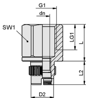
Конструктивные данные SC-A 055-AR G3/8-IG L
