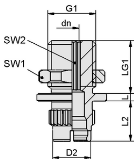
Dati di costruzione SC-A 055-AR G1/4-AG L
