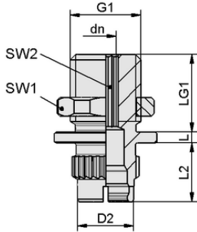
Tasarım verileri SC-A 055-AR G1/4-AG L
