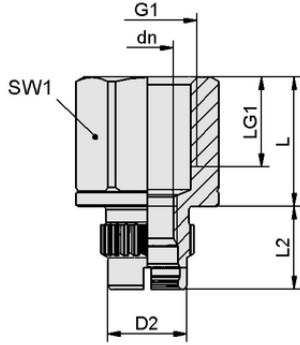
Tasarım verileri SC-A 055-AR G1/4-IG L
