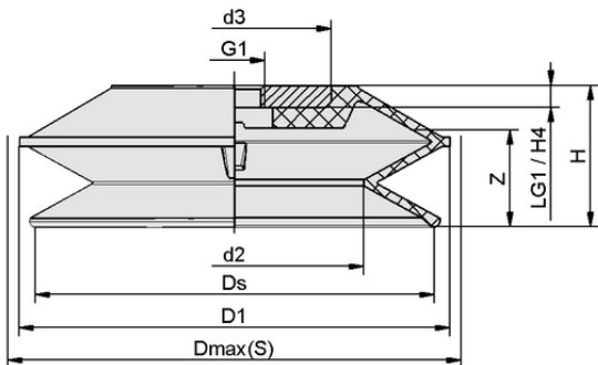
Datos de diseño FSGPL 120 HT1-60 G1/2-IG
