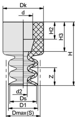
Données de construction FG 9 SI-HD-65 N016
