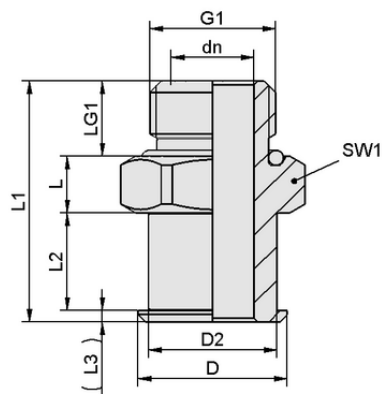
Datos de diseño SC 080 G1/8-AG
