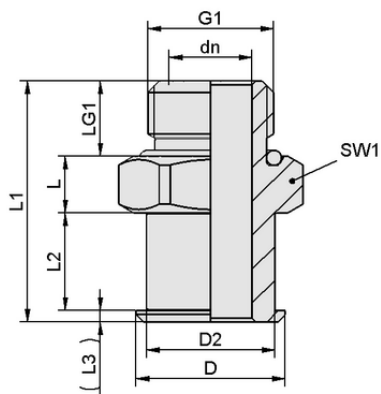
Конструктивные данные SC 080 G1/8-AG
