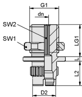
Design data SC-A 045-AR M10-AG L
