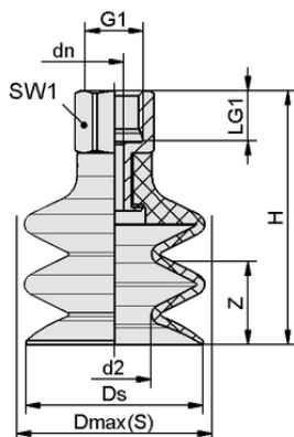
デザインデータ FSG 4 NBR-CO-55 M5-IG
