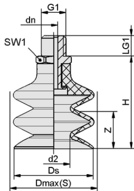
デザインデータ FSG 4 NBR-CO-55 M5-AG
