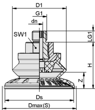
Datos de diseño SAB 125 HT1-60 G3/8-AG
