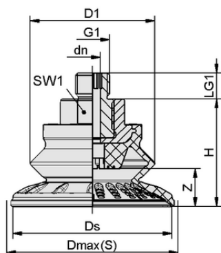
デザインデータ SAB 60 HT1-60 G1/4-AG
