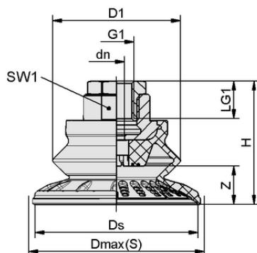
Конструктивные данные SAB 30 HT1-60 G3/8-IG
