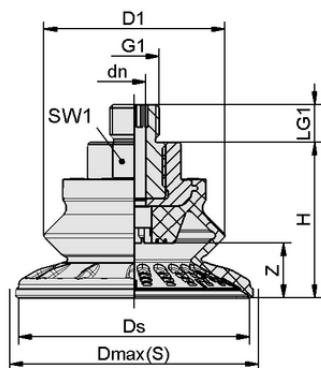
Конструктивные данные SAB 30 HT1-60 G3/8-AG
