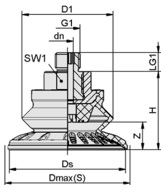
Конструктивные данные SAB 22 HT1-60 G3/8-AG
