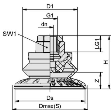
Dati di costruzione SAB 22 HT1-60 G3/8-IG
