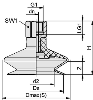
デザインデータ FSGA 6 NBR-55 M5-IG
