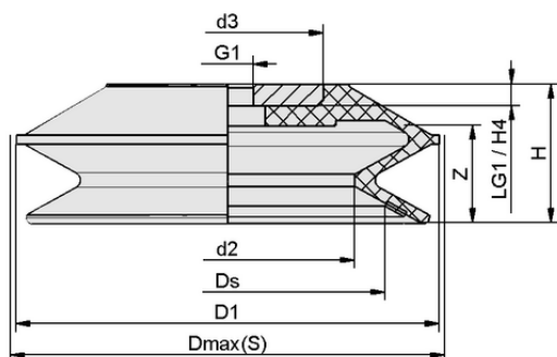
デザインデータ FSGPL 120 NBR-55 G1/2-IG DR
