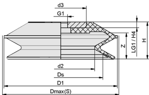
Dati di costruzione FSGPL 120 NBR-55 G1/2-IG DR
