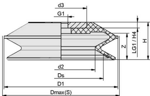
デザインデータ FSGPL 200 NBR-55 G1/2-IG DR
