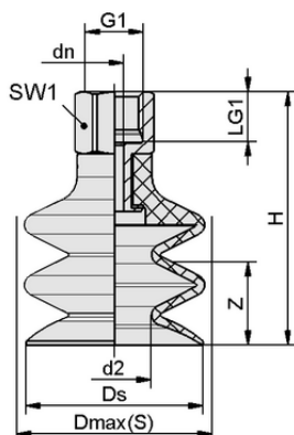
Конструктивные данные FSG 4 NBR-55 M5-IG
