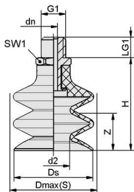
デザインデータ FSG 4 NBR-55 M5-AG
