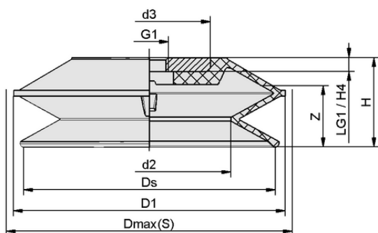
Конструктивные данные FSGPL 120 NBR-55 G1/2-IG
