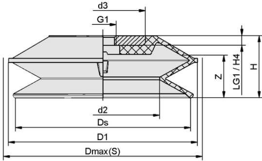
Tasarım verileri FSGPL 120 NBR-55 G1/2-IG
