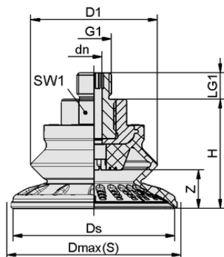
Datos de diseño SAB 100 HT1-60 G1/4-AG
