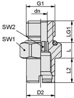
Tasarım verileri SC-A 065 M14x1.5-AG L
