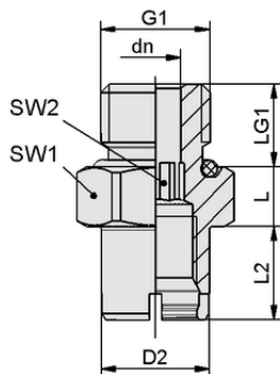
Design data SC-A 045 M14x1.5-AG L
