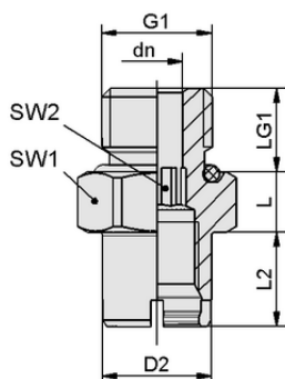
Datos de diseño SC-A 045 M10-AG L
