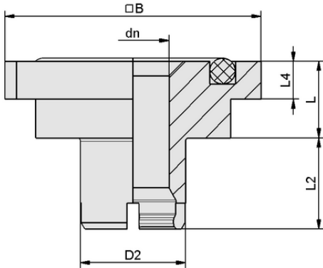
Tasarım verileri SC-A 055 RA L
