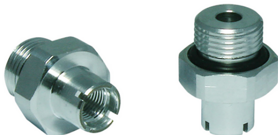
SC-A 055 G3/8-AG L
